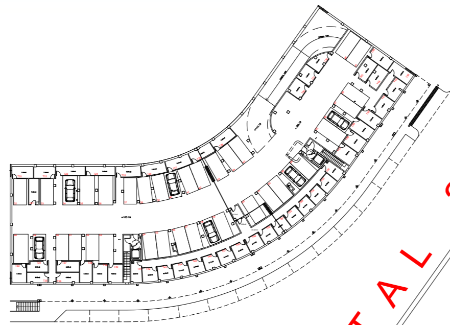
PLANTA SÓTANO -1
