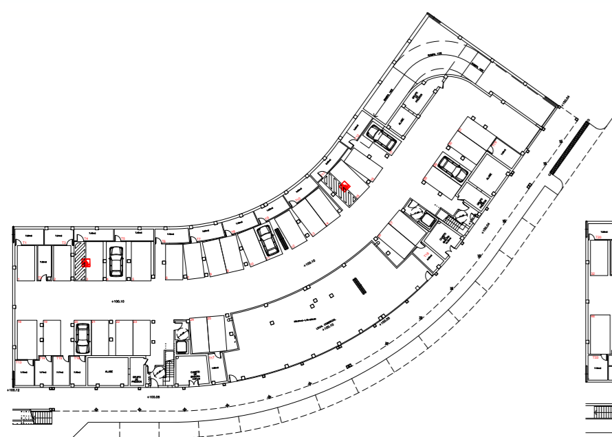
PLANTA SÓTANO -2
